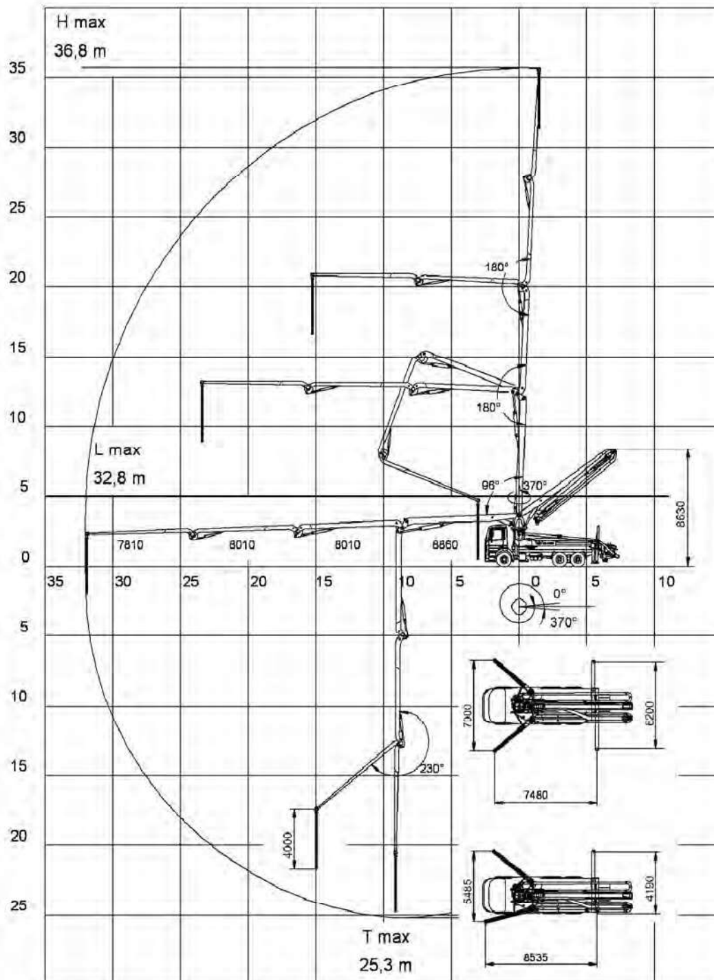
Abb. 3.6 Reichweitendiagramm 37 R 4 XXH
